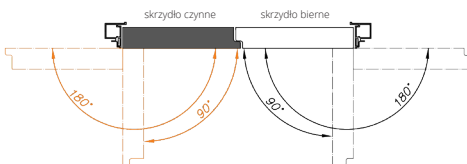
C. Drzwi lewe otwierane na zewnątrz
