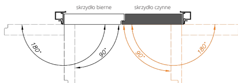
D. Drzwi prawe otwierane na zewnątrz
